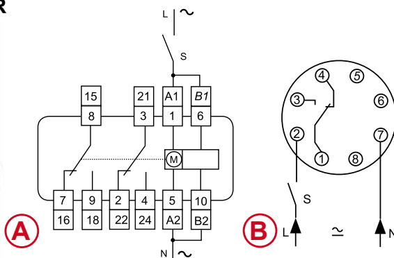
Funktion 16: anzugsverzögert mit Sofortkontakt
