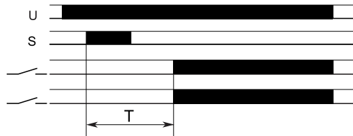
Funktion 34: 2 Relais Blinkgeber pausenbeginnend nach Impuls
