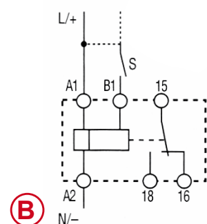
Funktion 3: Blinkgeber (impulsbeginnend)
