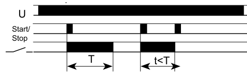
Funktion 38: Anzugsverzögert mit Start/Stop Taste
