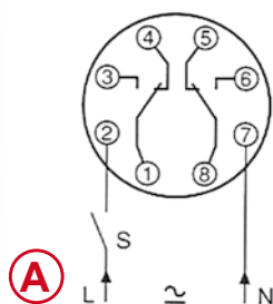
Funktion 18: Einschaltwischer (2 Relais)
