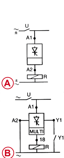
Funktion 1: Anzugsverzögerung
