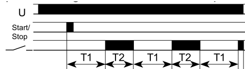
Funktion 41: Impulsgeber mit Start/Stop Taste
