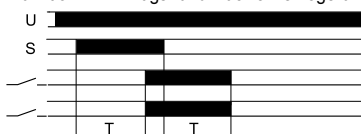
Funktion 25: Impulsformer (2 Relais)
