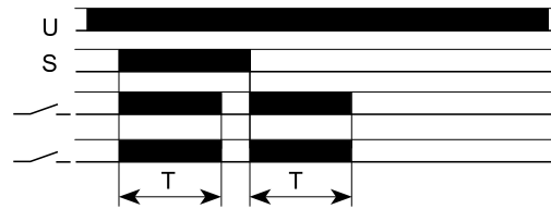
Funktion 37: Rückfallverzögert mit Start/Stop Taste
