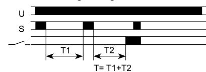
Funktion 9: anzugsverzögert, additiv
