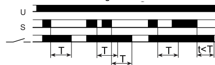
Funktion 2: rückfallverzögert mit Steuerkontakt
