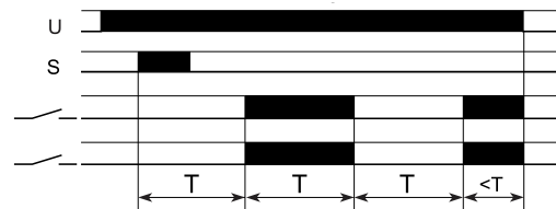
Funktion 35: 2 Relais Blinkgeber impulsbeginnend nach Impuls
