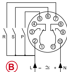
Funktion 20: Impulsgeber (2 Relais)
