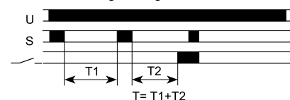
Funktion 10: einschaltwischend, additiv
