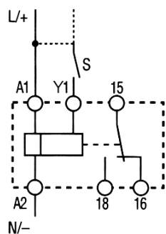
Funktion 4: Einschaltwischer
