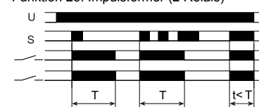
Funktion 25: Impulsformer (2 Relais)
