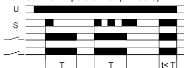
Funktion 33: 2 Relais anzugsverzögert nach Impuls
