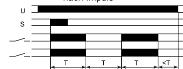
Funktion 36: Wischrelais (2 Relais)
