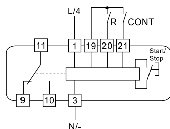
Funktion 39: Blinkgeber, impulsbbeginnend mit Start/Stop Taste
