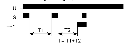
Funktion 10: einschaltwischend, additiv
