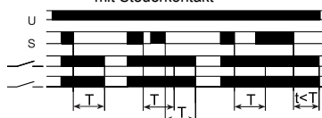
Funktion 24: Anzugs- und Rückfallverzögerung (2 Relais)
