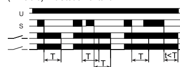
Funktion 22: Rückfallverzögerer (2 Relais) mit Steuerkontakt
