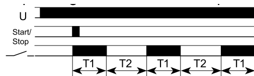
Funktion 40: Blinkgeber, pausenbeginnend mit Start/Stop Taste
