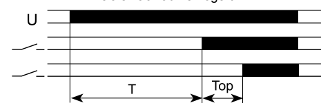
Funktion 27:1 Relais anzugsverzögert 1 Relais nachlaufverzögert
