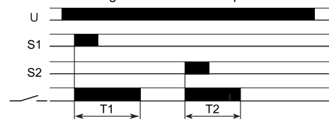
Funktion 32: Taktgeber - Start nach Impuls
