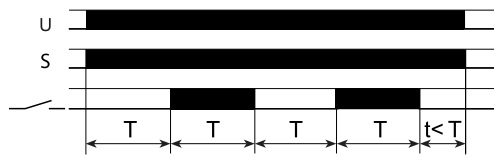
Funktion 32: Taktgeber - Start nach Impuls
