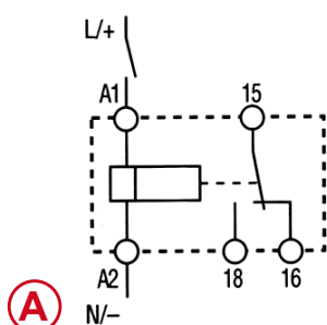
Funktion 1: Anzugsverzögerung
