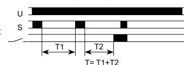
Funktion 10: einschaltwischend, additiv
