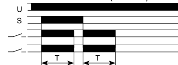
Funktion 36: Wischrelais (2 Relais)
