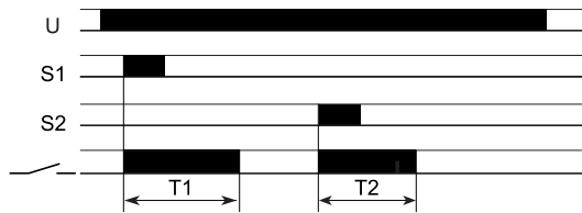
Funktion 33: 2 Relais anzugsverzögert nach Impuls
