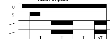
Funktion 34: 2 Relais Blinkgeber pausenbeginnend nach Impuls
