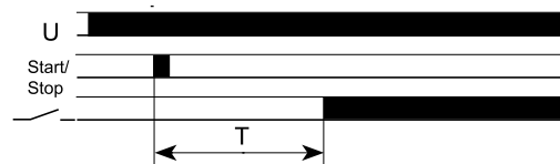
Funktion 39: Blinkgeber, impulsbbeginnend mit Start/Stop Taste
