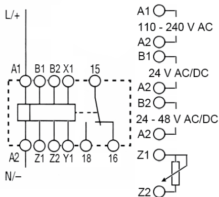
Funktion 2: rückfallverzögert mit Steuerkontakt
